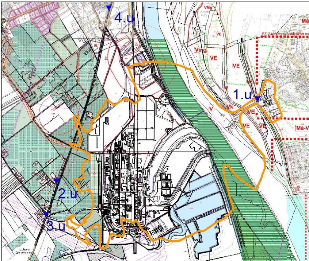
77. ábra: Az üzemi területi építés összesített hatásterülete
