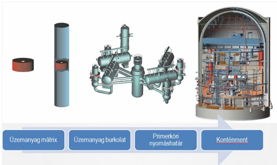
8. ábra: Mérnöki gátak atomerőművi blokkoknál [7]
