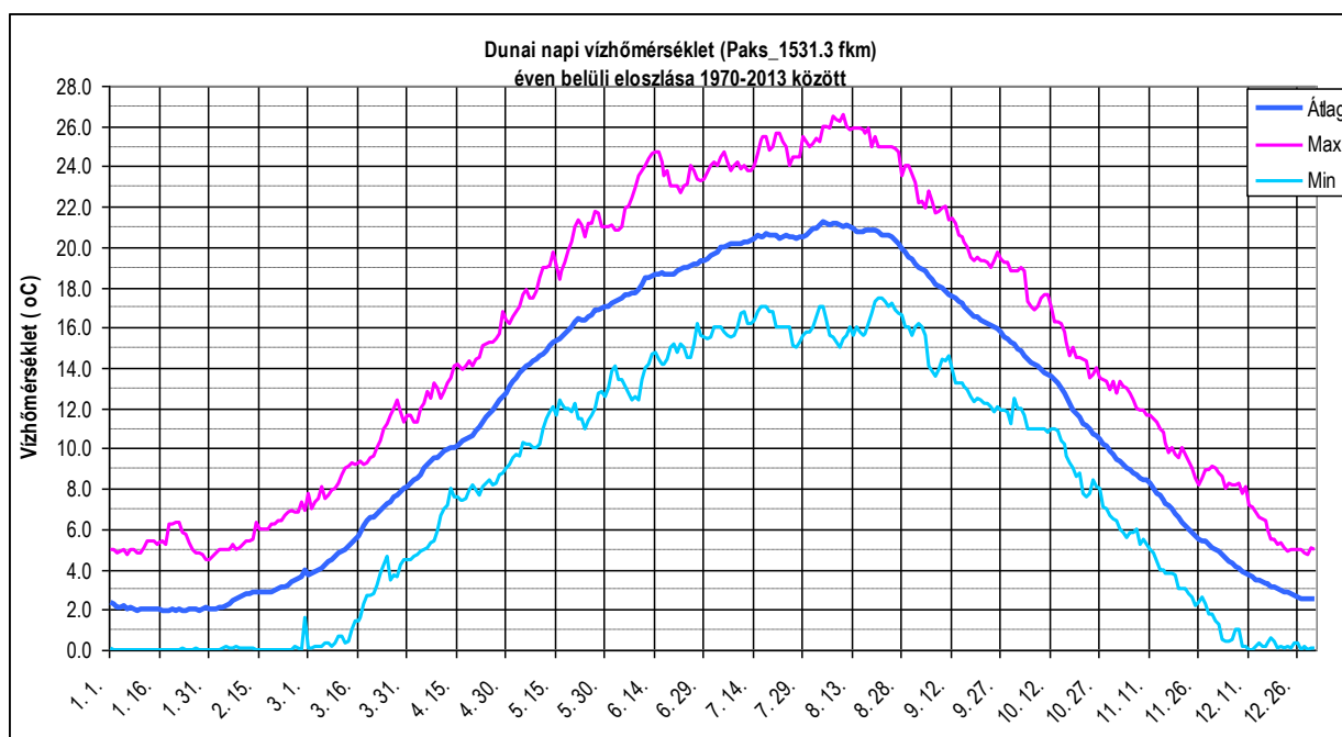
73. ábra: Dunai napi víz hőmérséklet (Paks) éven belüli eloszlás vizsgálata 1970-2013. között
