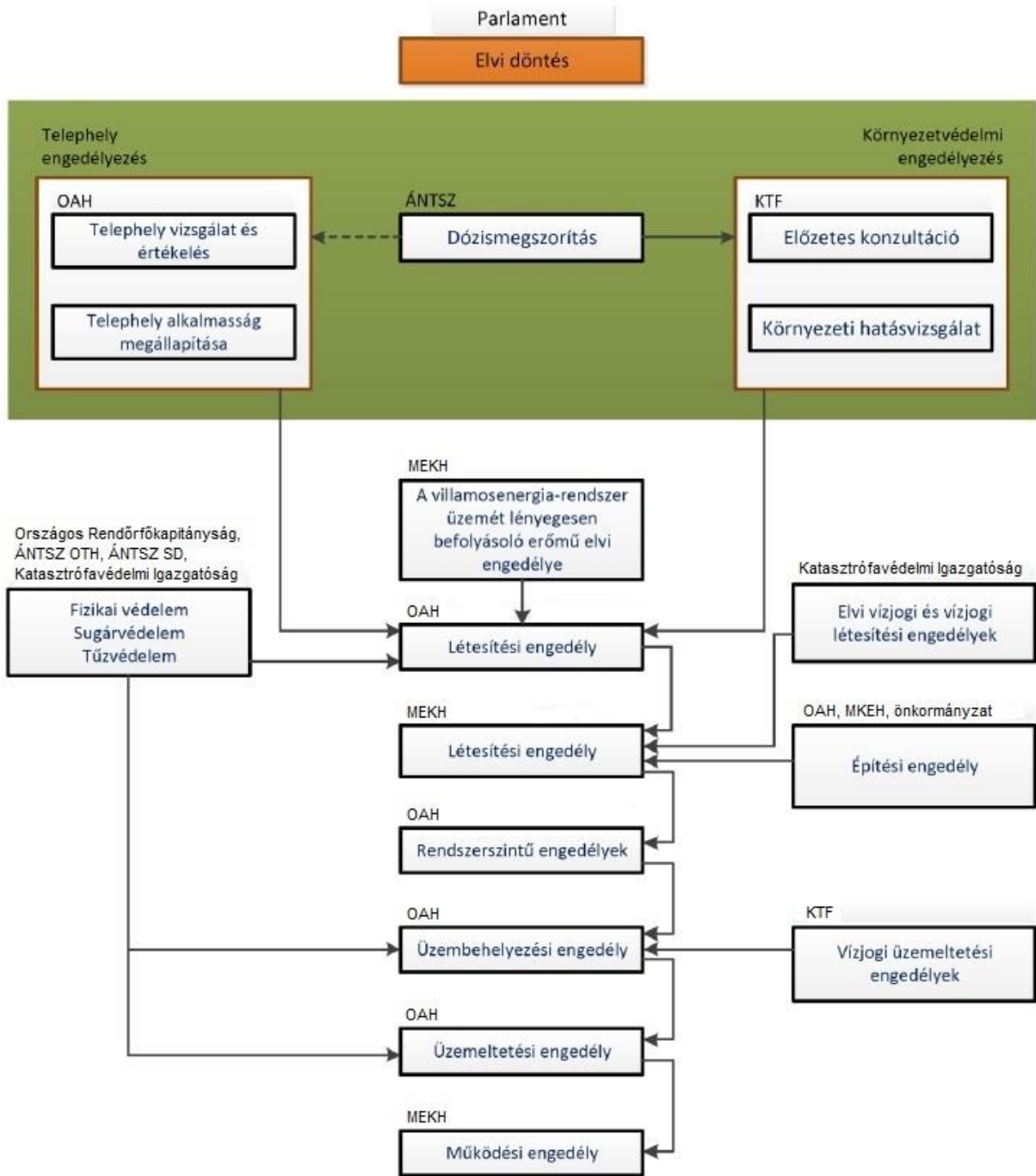
1. ábra: Atomerőmű engedélyztetésének folyamata
