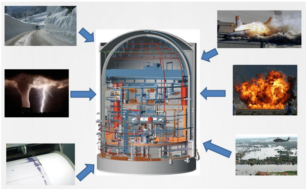
10. ábra: A külső konténment védelmet ad a külső hatásokkal szemben [7]
