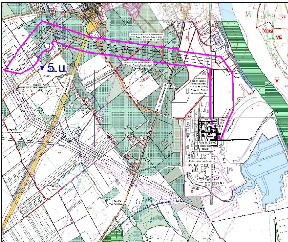
78. ábra: Távfvezeték-építés összesített hatásterülete
