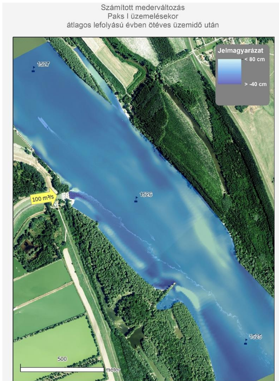
61. ábra: Számított Duna mederváltozások 5 év üzemelés után, 2\,300 \text{ m}^3/\text{s} -os dunai hozam (átlagos hidrológiai év) és 100 \text{ m}^3/\text{s} -os hűtővíz-kivétel esetén – Paksi Atomerőmű önálló üzemelése (2014-2025)
