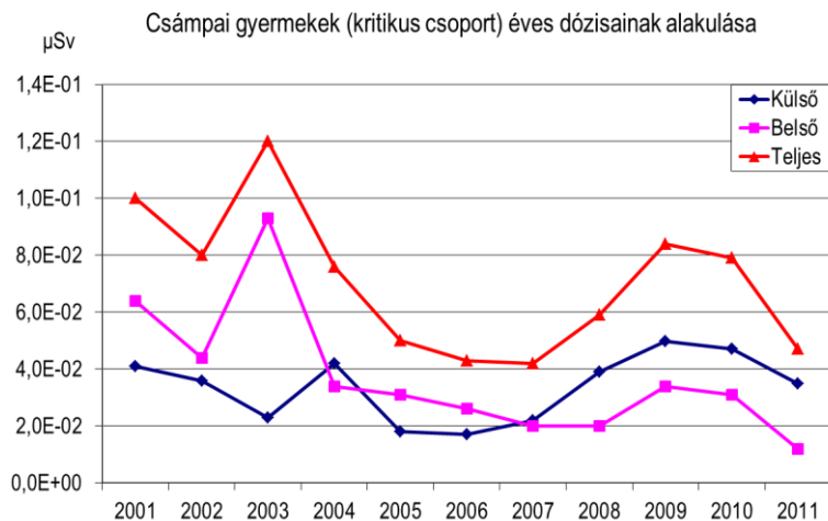
101. ábra: Csámpai gyermekek (kritikus csoport) éves dózisainak alakulása az erőművi kéménykibocsátásokból
