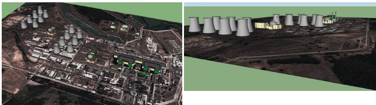
28. ábra: Természetes huzatú nedves hűtőtornyos, 100 m-re korlátozott magassággal - látványterv (madártávlat és oldalnézet)
