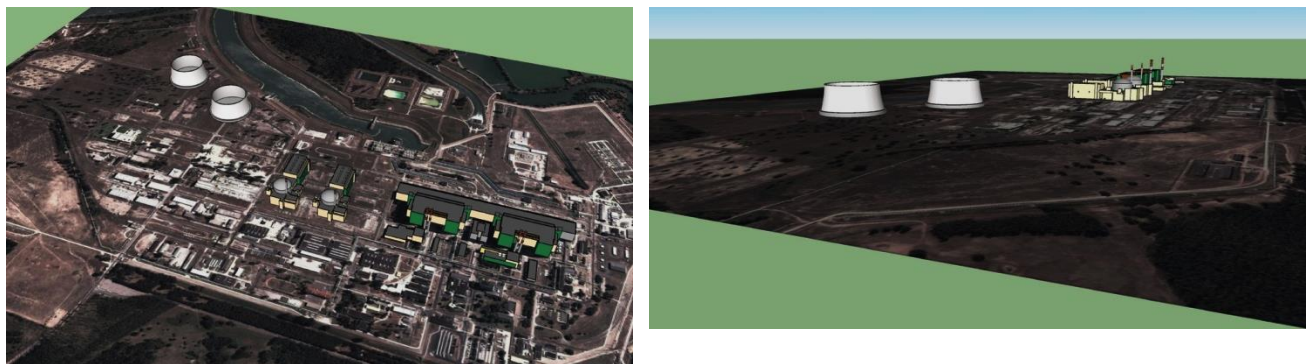
29. ábra: Természetes huzatú nedves hűtőtornyos ventilátoros rásegítéssel - látványterv (madártávlat és oldalnézet)
