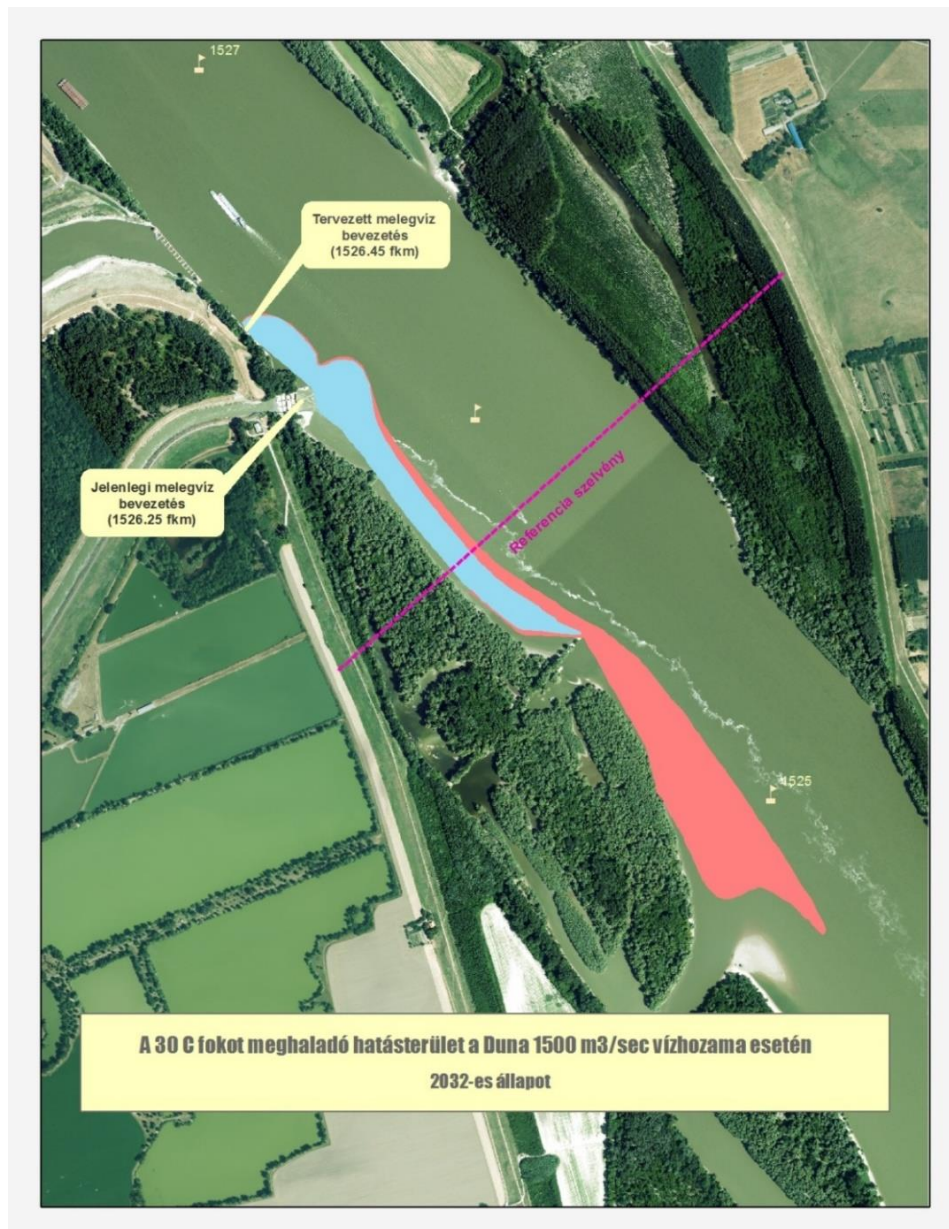
65. ábra: A hőcsóva 30 °C feletti hatásterülete – 2032. évi állapot ( T_{Duna,max}=26,38^{\circ}\text{C} , Q_{Duna}=1500\text{ m}^3/\text{s} , melegvíz hozam: 100\text{ m}^3/\text{s} + 132\text{ m}^3/\text{s} )
