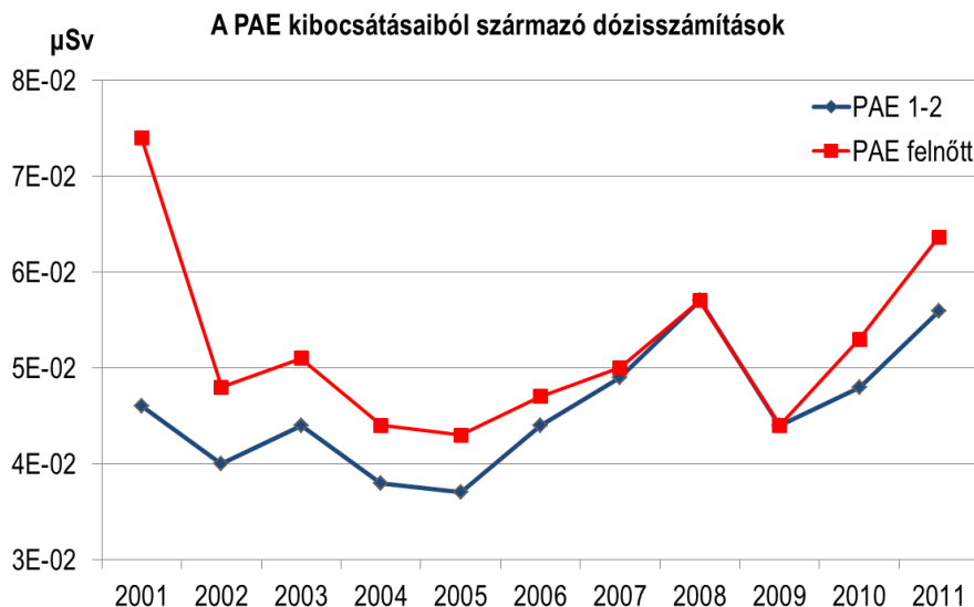
102. ábra: A Paksi Atomerőmű folyékony kibocsátásából származó sugárterhelések a gerjени gyermek (1-2 éves) és felnőtt korcsoportokra vonatkozóan
