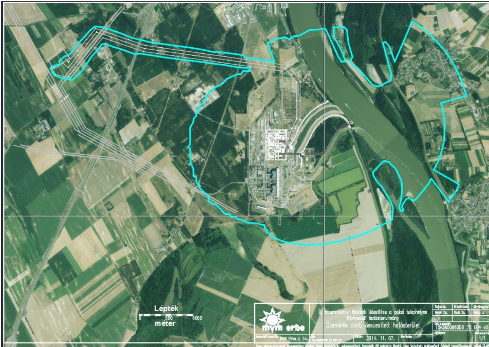
107. ábra: Paks II üzemelésének összesített hatásterülete
