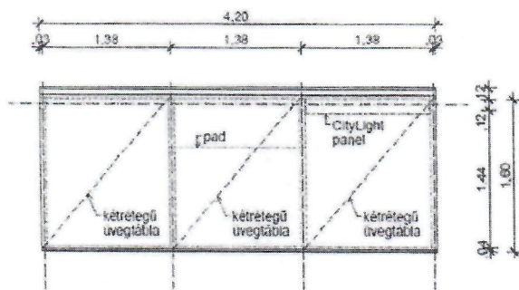
FELÖLNÉZET
