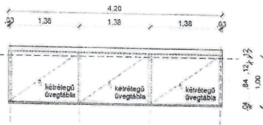
FELÜLNÉZET
