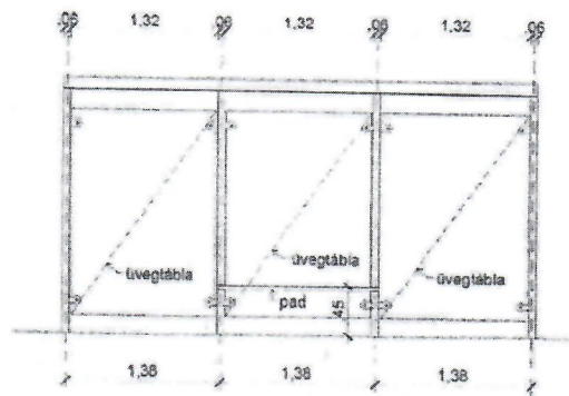
ELŐLNÉZET
