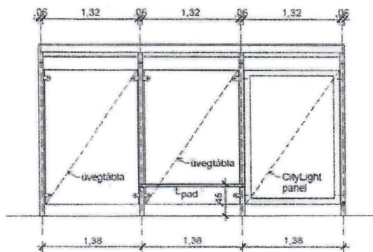
ELÖLNÉZET
