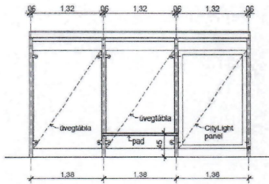
ELŐLNÉZET
