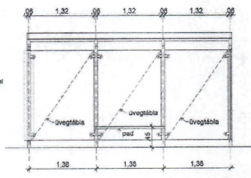
ELÖLNÉZET
