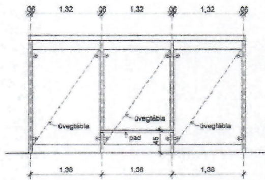
ELŐLNÉZET
