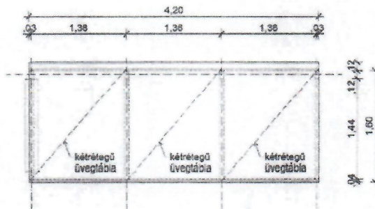
FELÜLNÉZET
