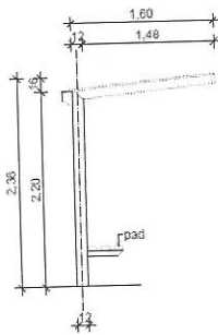
BAL OLDALI NÉZET
