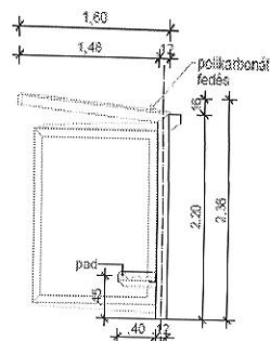
JOBB OLDALI NÉZET
